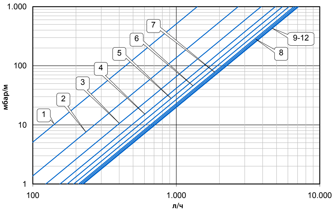
Диаграмма гидравлических потерь коллектора в зависимости от количества выходов (в открытом состоянии)
